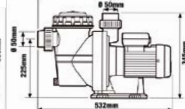
NXP75, NXP100 et NXP150
